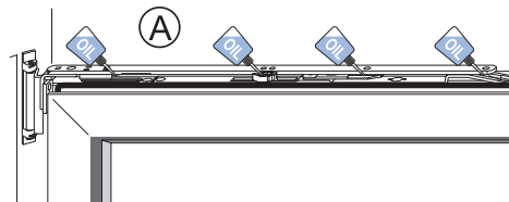
Bild 4: Schere
