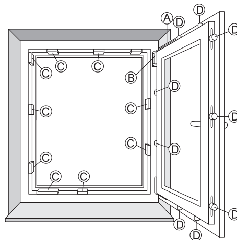
Bild 1: Schmierstellenübersicht
